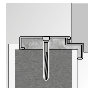
OPAL Montaż na dyble.
