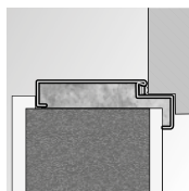
AGAT montaż bez dodatkowych elementów kotwiących
