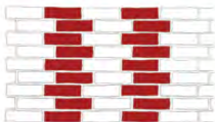
Wiązanie wozówkowe - przesunięcie o 1/4 cegły
