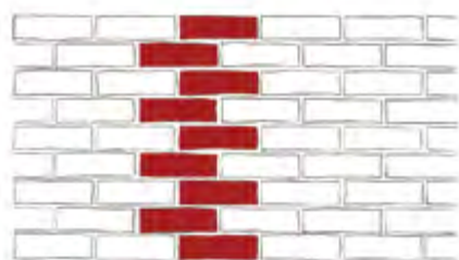
Wiązanie wozówkowe - przesunięcie o 1/2 cegły
