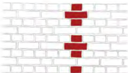
Wiązanie krzyżowe typ I
